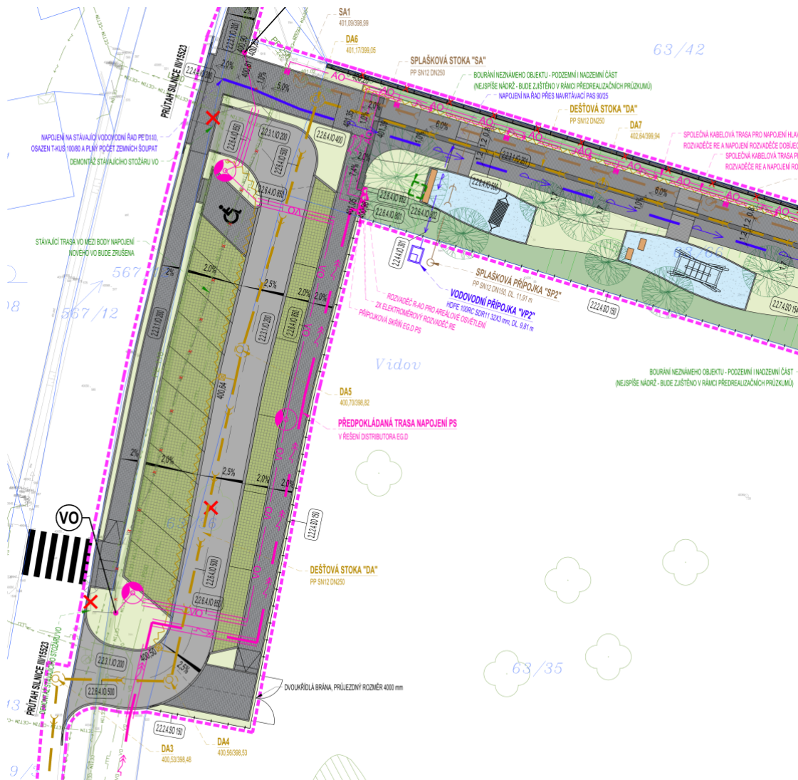
výřez z připravovaného projektu základní školy
